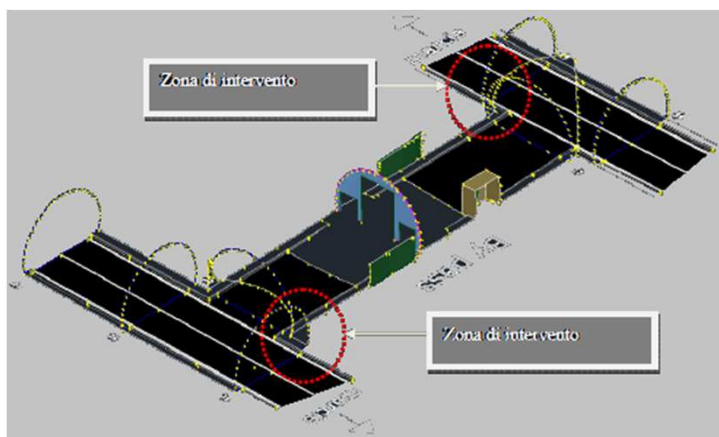
Progetto - Tipologico protezione spigoli dei By-pass
